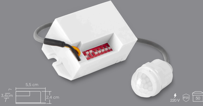
ZMR-537 MİNİ RADAR SENSÖR
