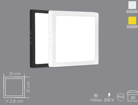
ZMR-246 18W ALÜ. KARE SIVA ÜSTÜ PANEL
