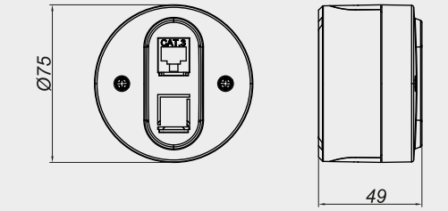
NUMERİS TELEFON PRİZİ CAT3
