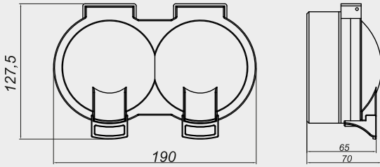
W.P. KOMÜTATÖR + TOPRAKLI PRİZ
