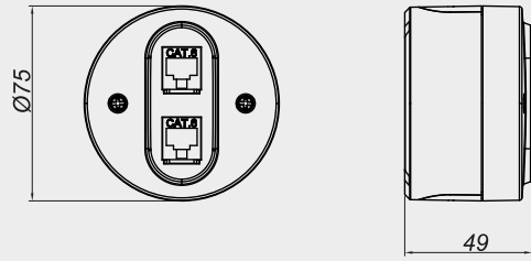
İKİLİ DATA PRİZİ CAT6
