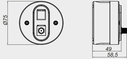
UYDU F CONNECTOR
