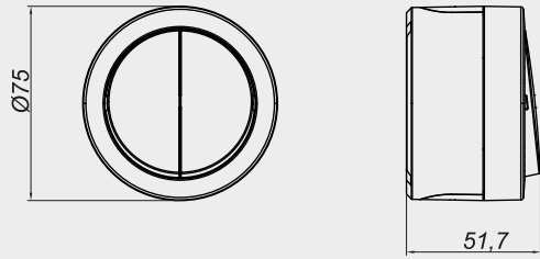
KOMÜTATÖR
