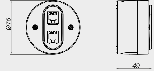
NUMERİS TELEFON PRİZİ CAT3 + DATA PRİZİ CAT6
