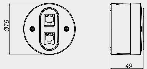
İKİLİ NUMERİS TELEFON PRİZİ CAT3
