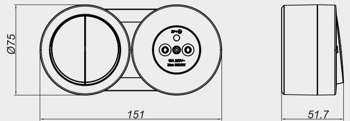
KOMÜTATÖR + UPS PRİZ
