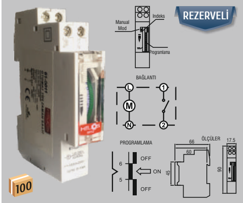
W Otomat Tipi Zaman Rölesi
