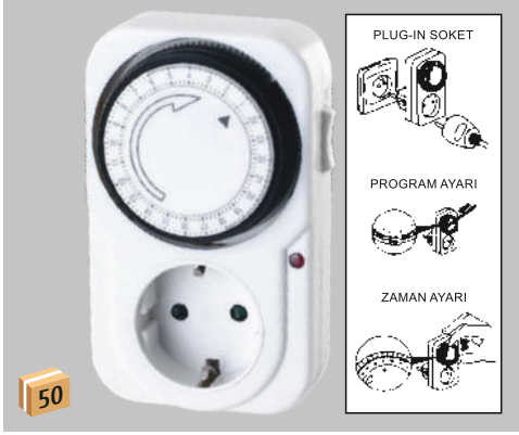
Mekanik Zaman Saati
