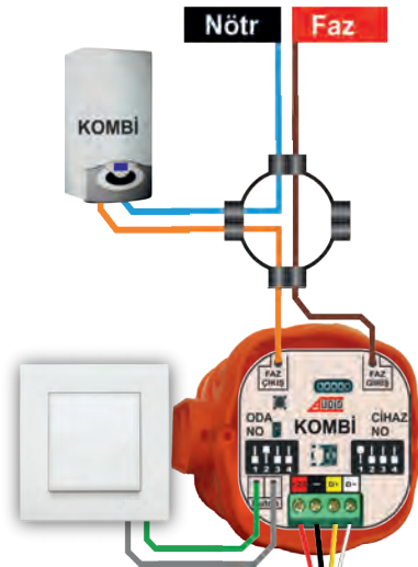
KOMBİ BAĞLANTISI
