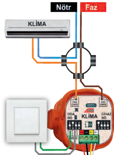
KLİMA BAĞLANTISI
